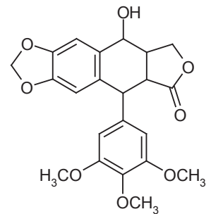
ポドフィロトキシン
