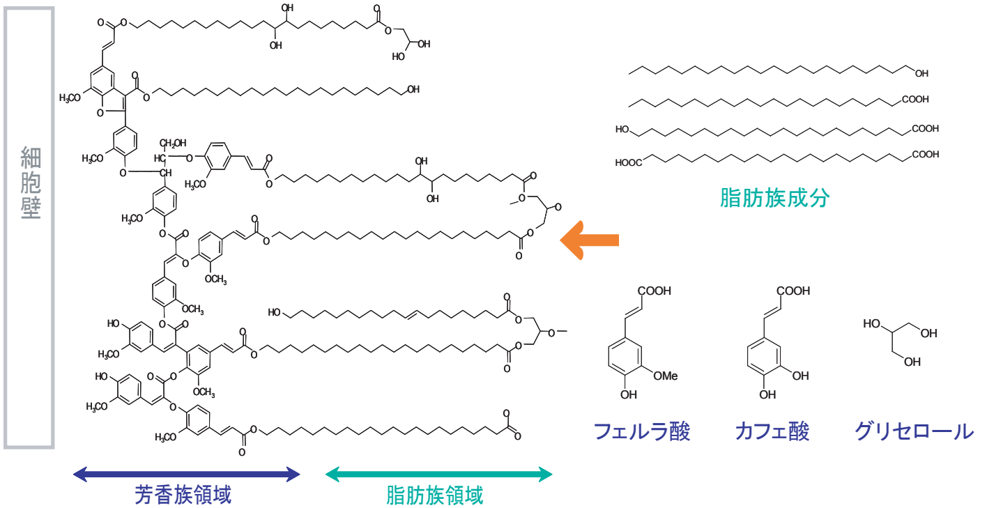
スベリンの予想構造図
