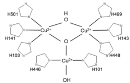
活性部位の原子モデル
