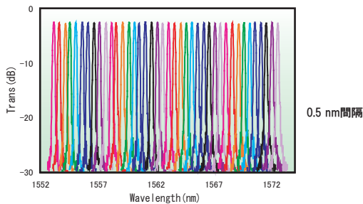
作製した40ch-FBGの反射スペクトルの例
