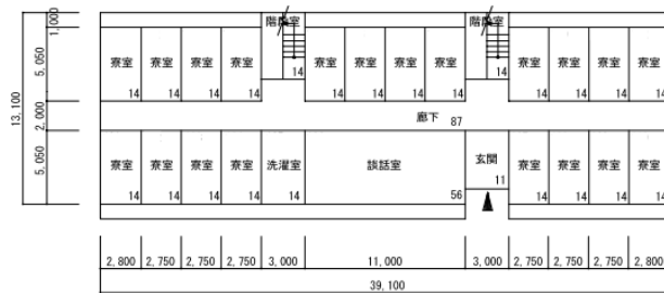
1階平面図
