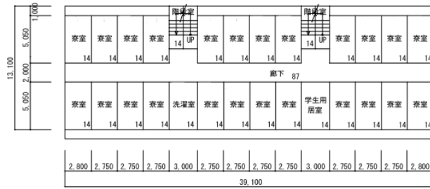
2, 3階平面図
