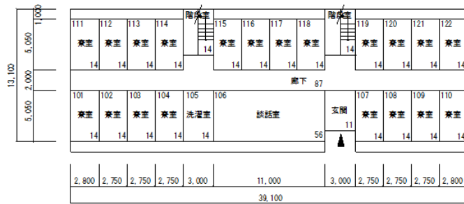
1階平面図
